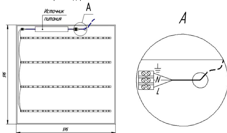
Рис.2 Светильник Офис Тендер 4x18
