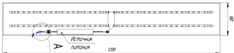
Рис.1 Светильник Офис Тендер 2x36
